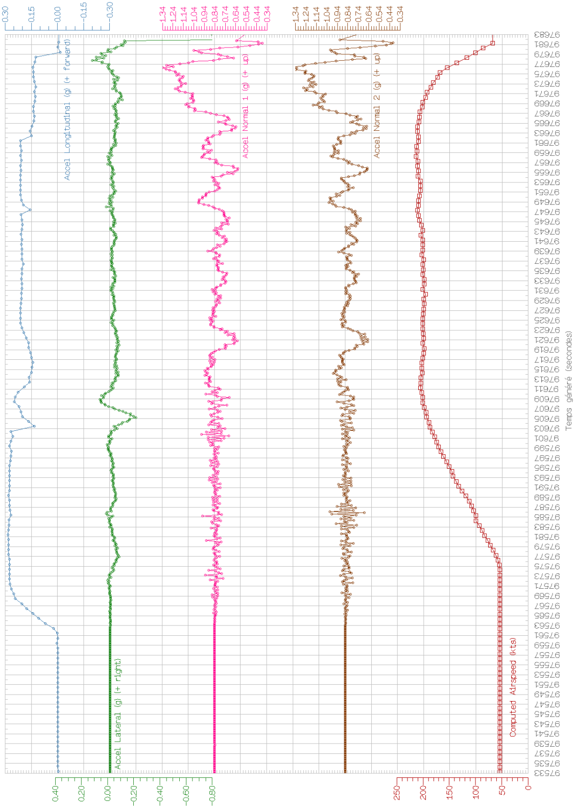
Planche 1: Accelerations/Evènement
